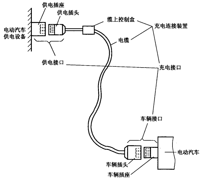
图 1 电动汽车传导充电用连接装置示意图
